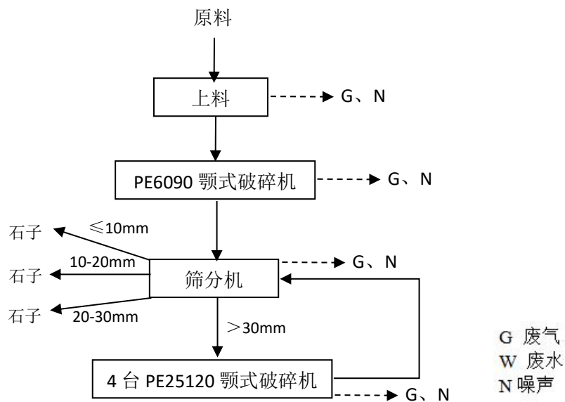
图 2-2 生产工艺流程及产污环节图
