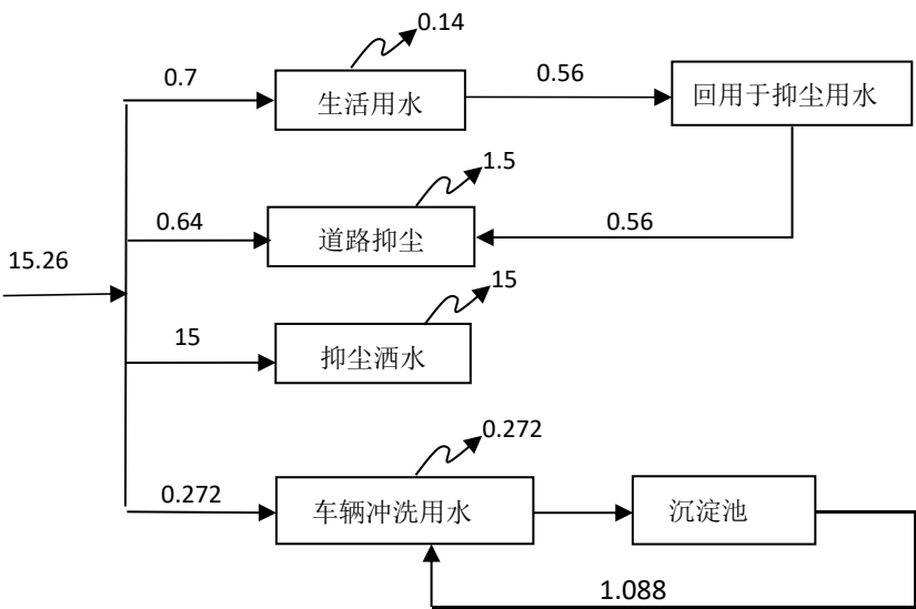
图 2-1 本项目营运期水平衡图（m 3 /d）
